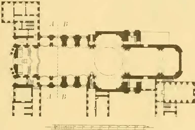
Fig. 77. Klosterkirche zu Zwiefalten, Grundriss A, des Obergeschoßes, B, des Erdgeschoßes.
